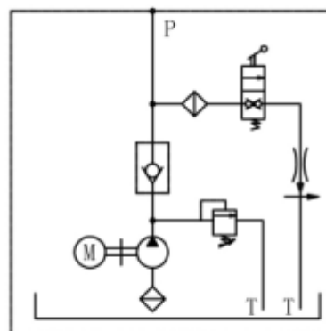
Сеть гидросистемы
