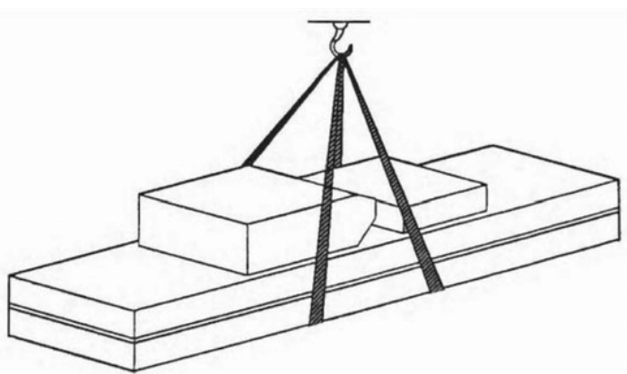
Рис.0. Строповка оборудования
